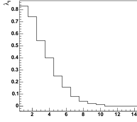
(d) Eigenvalues of Gram's matrix G
